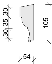
Det4 Akende ülemine karniis
