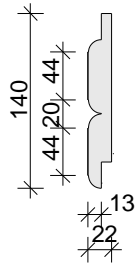
Det2 Vintsakapi vertikaalne voodrilaud
