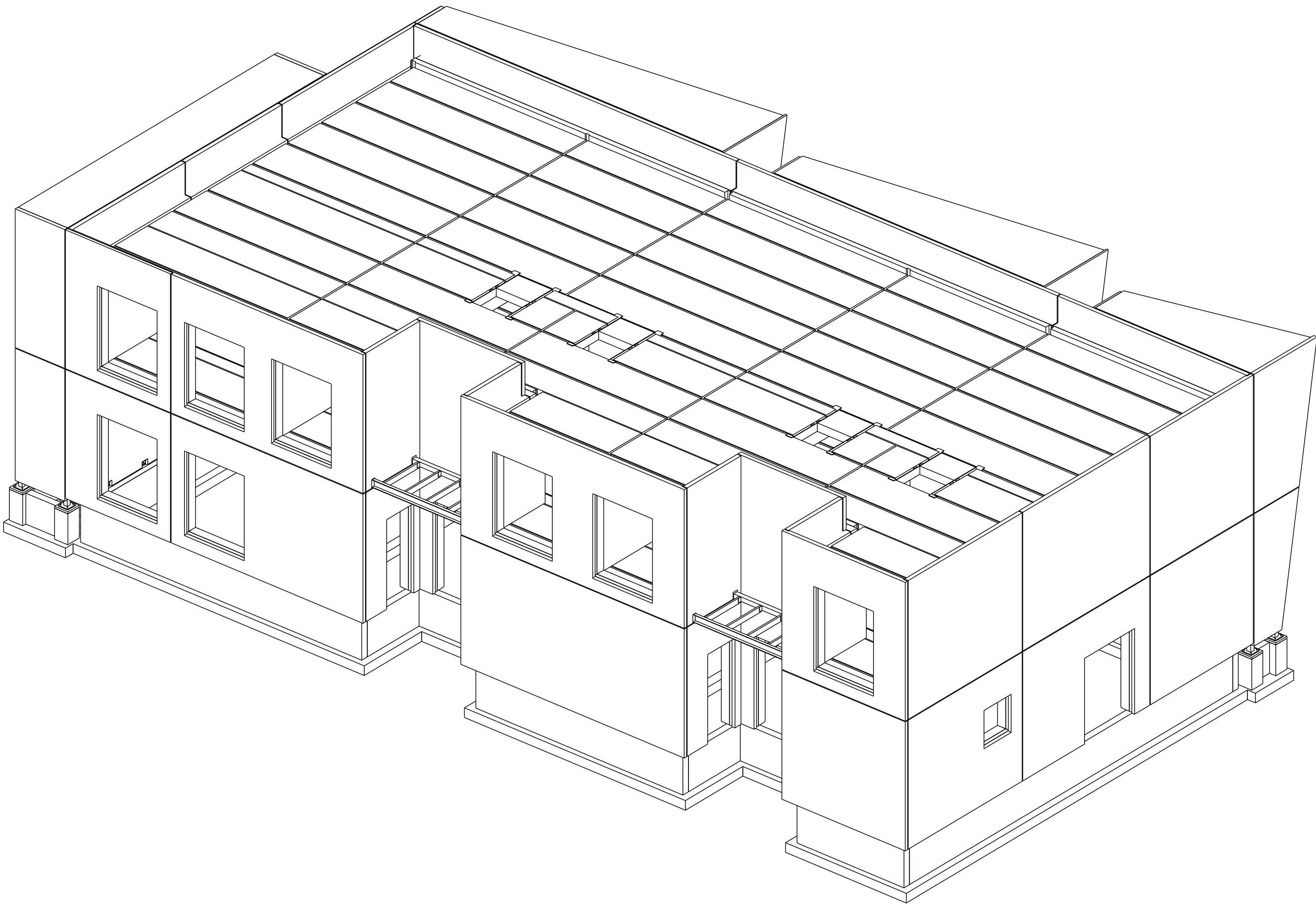
HOONE 3D VAADE TELJEST L-1 1:75
