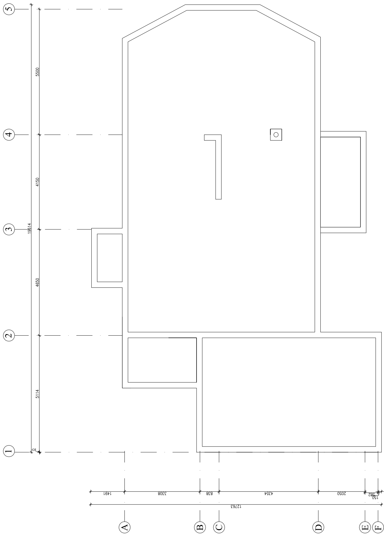
Rostvärkide plaan M 1:100
