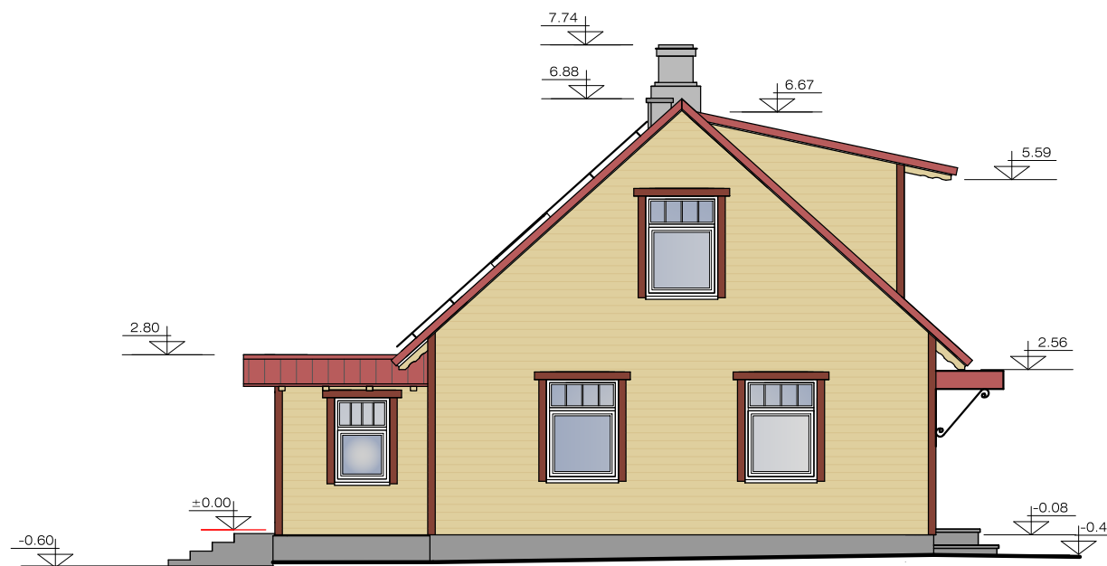
LÄÄNEPOOLNE OTSVAADE
