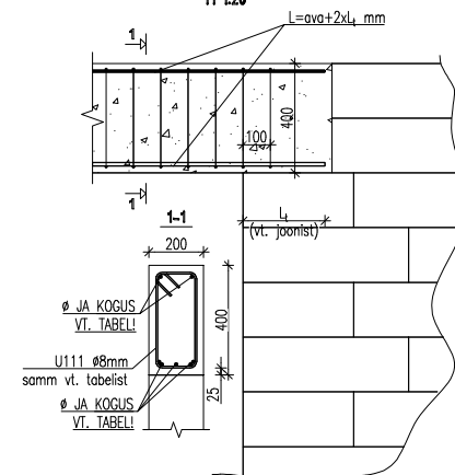
Silluse tüüplõige STL-01 M 1:20
