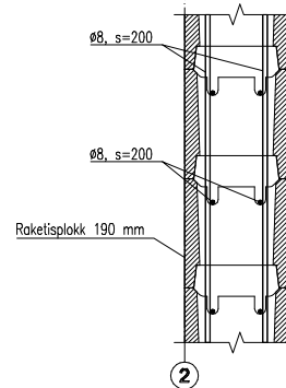
Selma lõige SL-01 M 1:10
