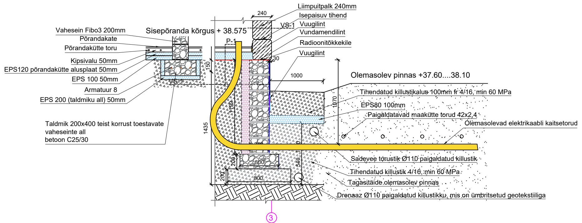
SOKLI SÄLM, VERTIKAALLÕIGE S-01
