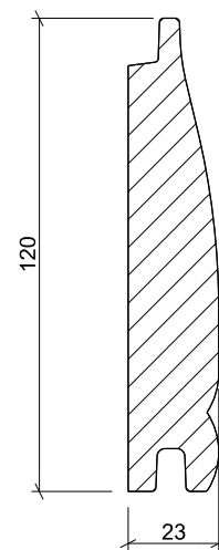
ORIGINAAL HORISONTAALNE FASSAADILAUD
