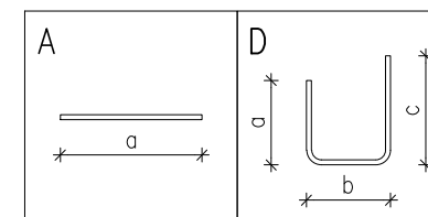
Sarruse painutustüübid
