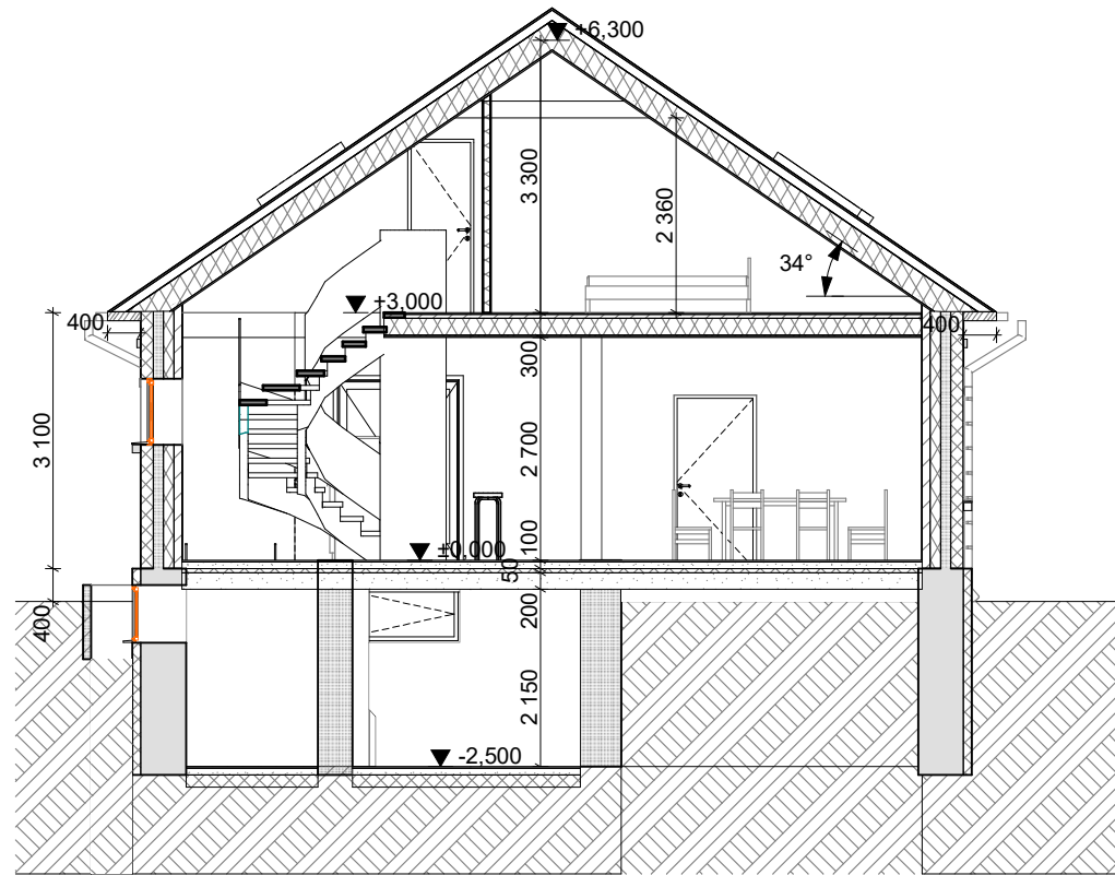
LÖIGE A-A
