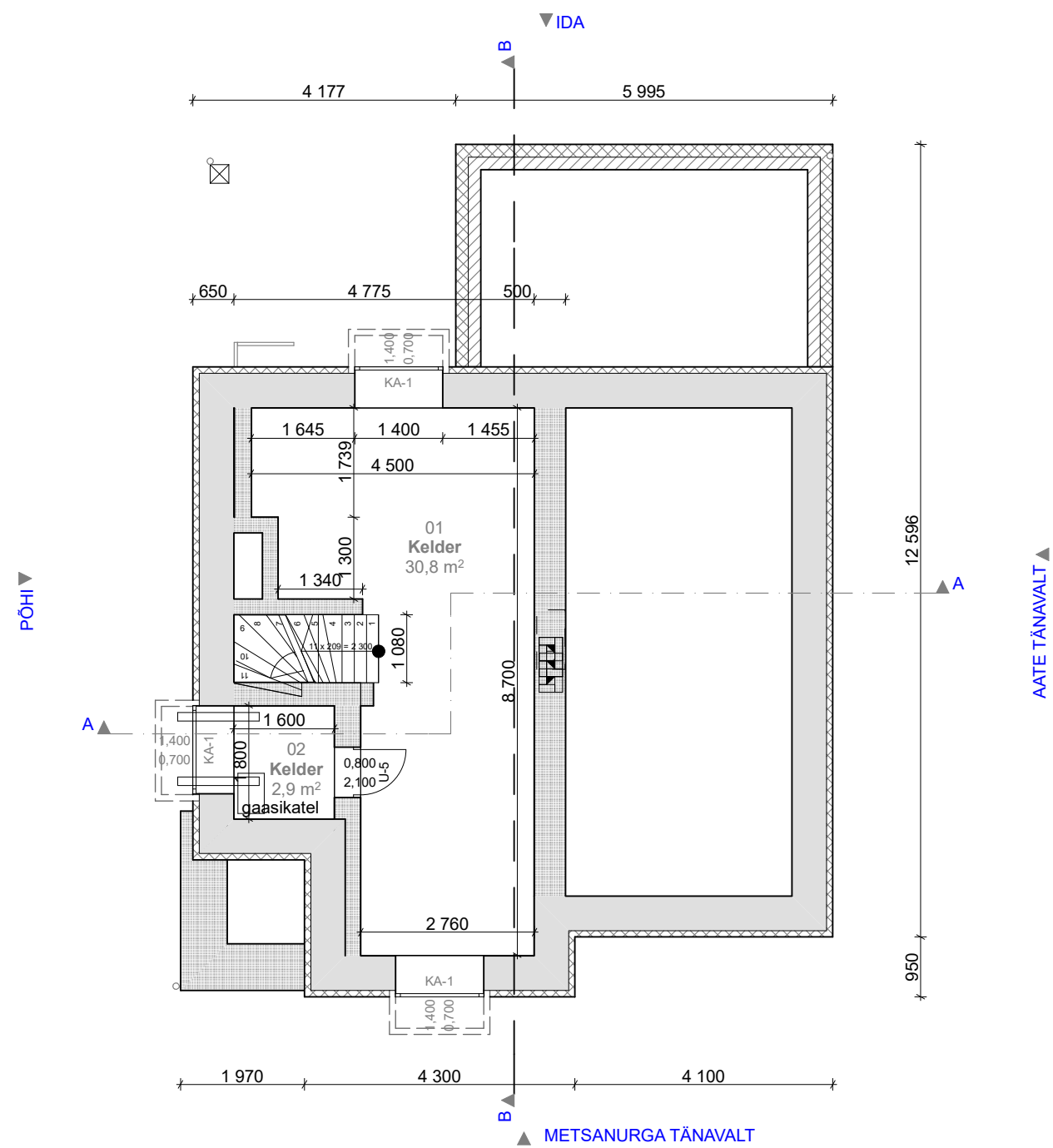
KELDRI PLAAN
