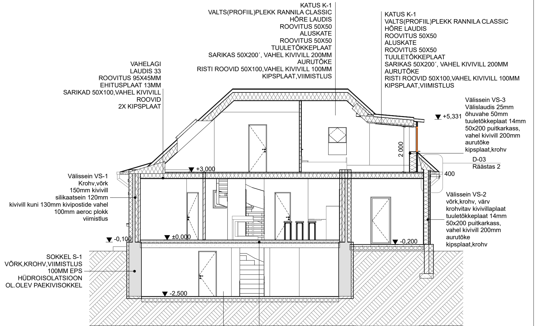
LÖIGE B-B
