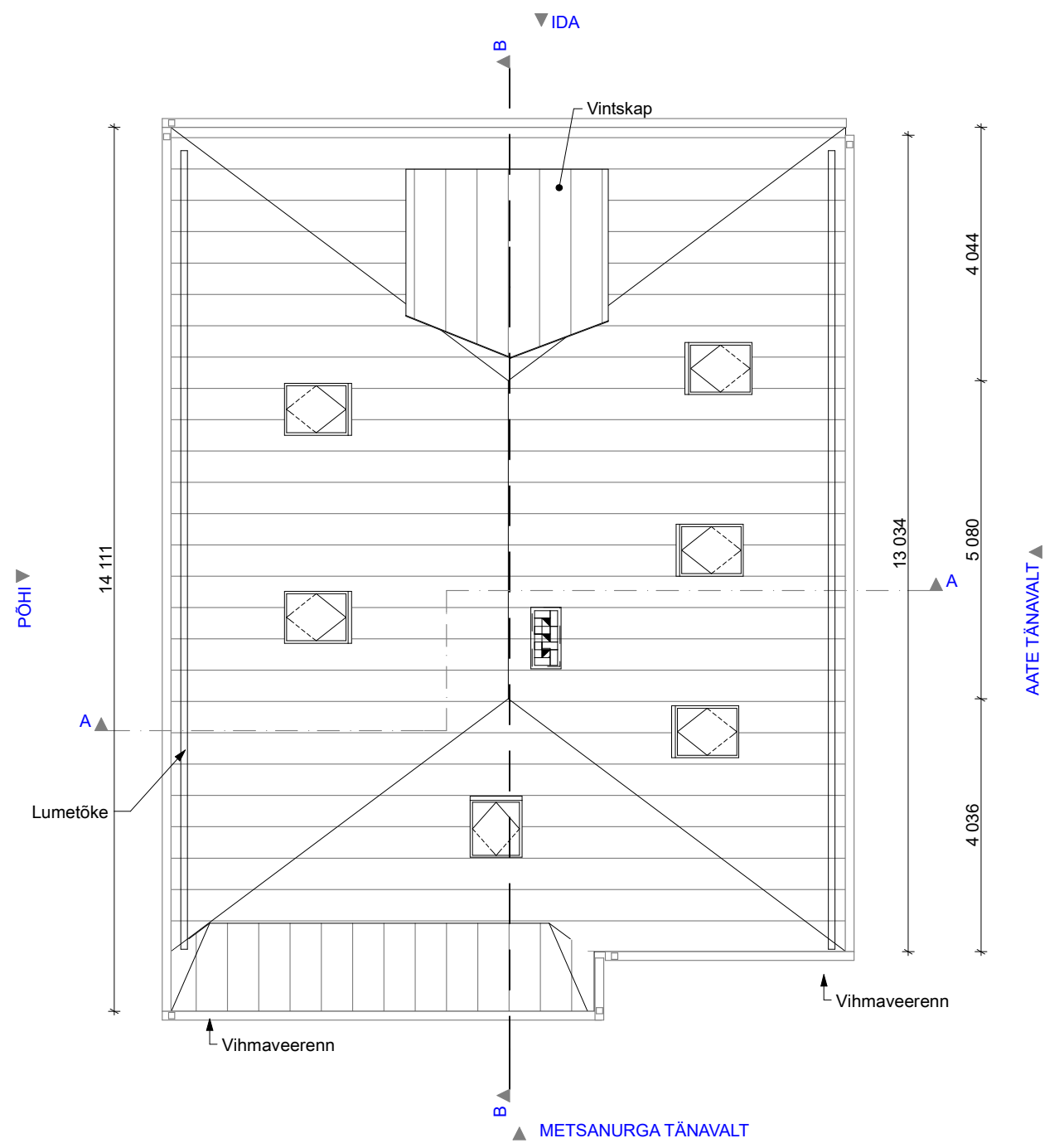
KATUSE PLAAN
