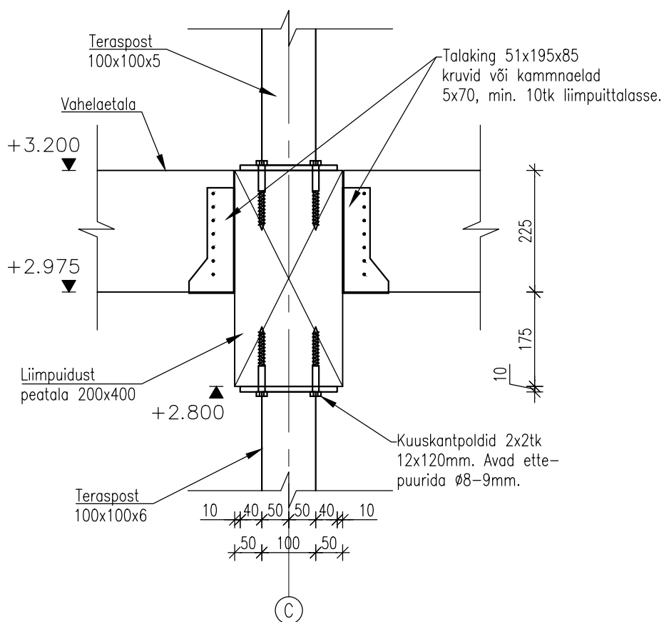
VL.det.-2 1:10
