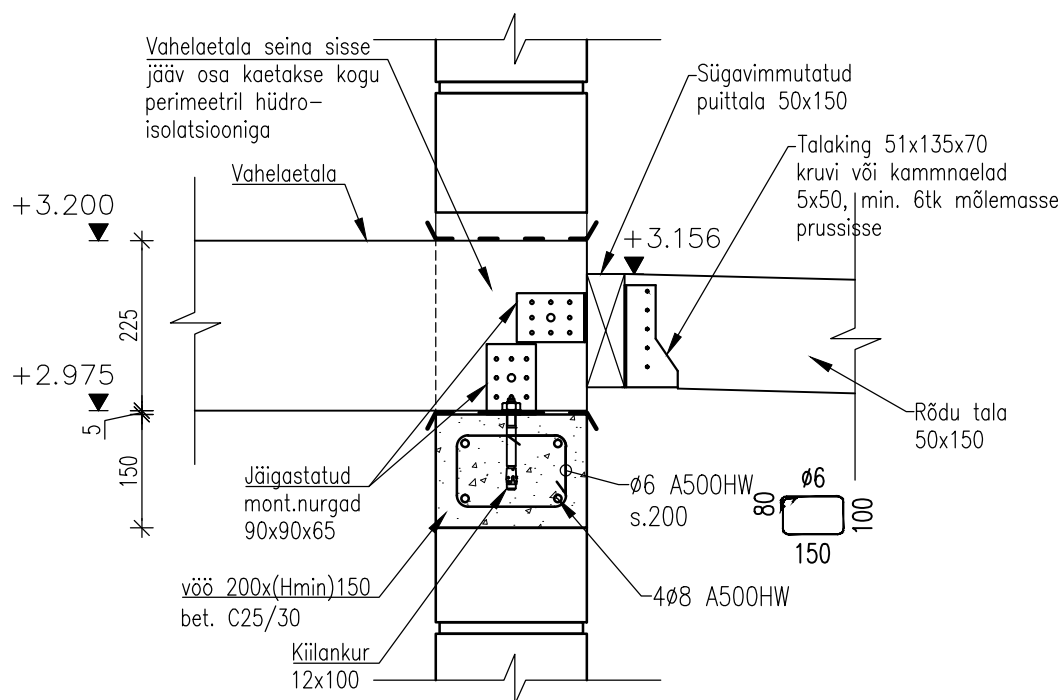
VL.det.-2 1:10
