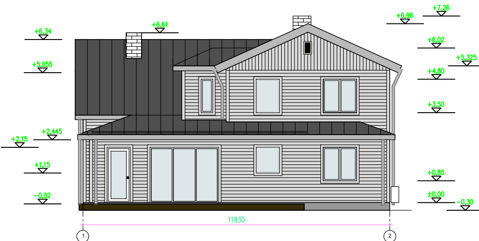
VAADE LÖUNAST
