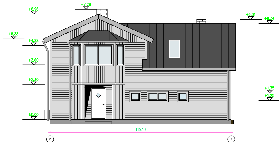
VAADE PÕHJAST
