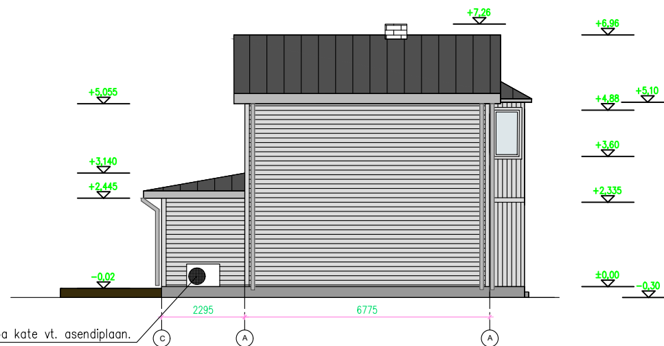
VAADE IDAST
