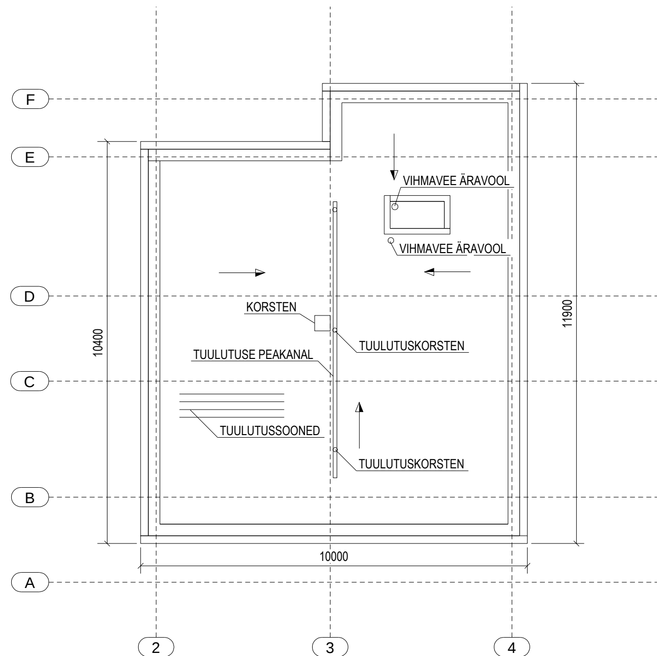
KATUSE PLAAN 1:100
