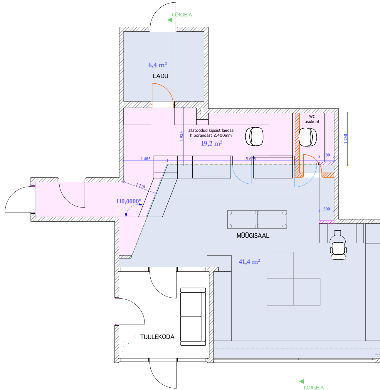
PLAAN
