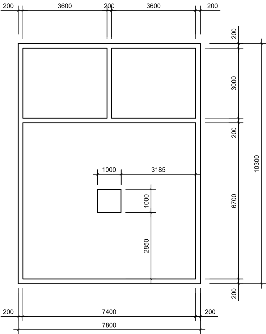
Vundament
