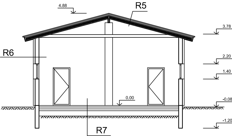
Lõige 1 - 1
