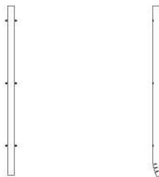
DET. 3 KAITSETORU VÕI -KARBIK VASTAVALT LÄBIMÕÕDULE
