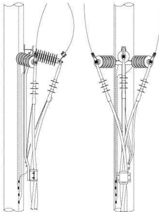
DET. 1 OTSAMUHVI KINNITUS PINGEPIIRIKUTEGA M 1:25
