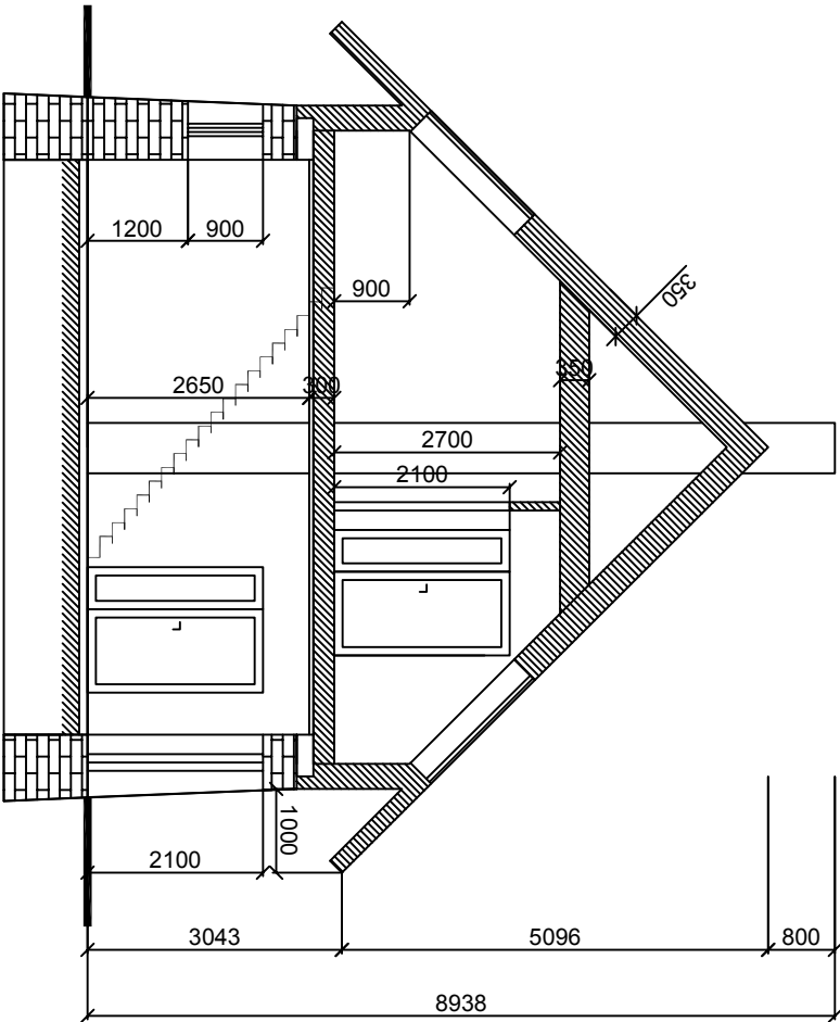
LÕIGE 1 - 1
