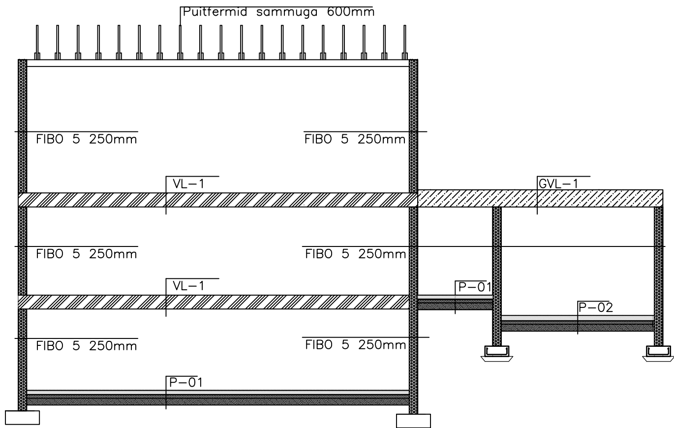
Lõige 1-1
