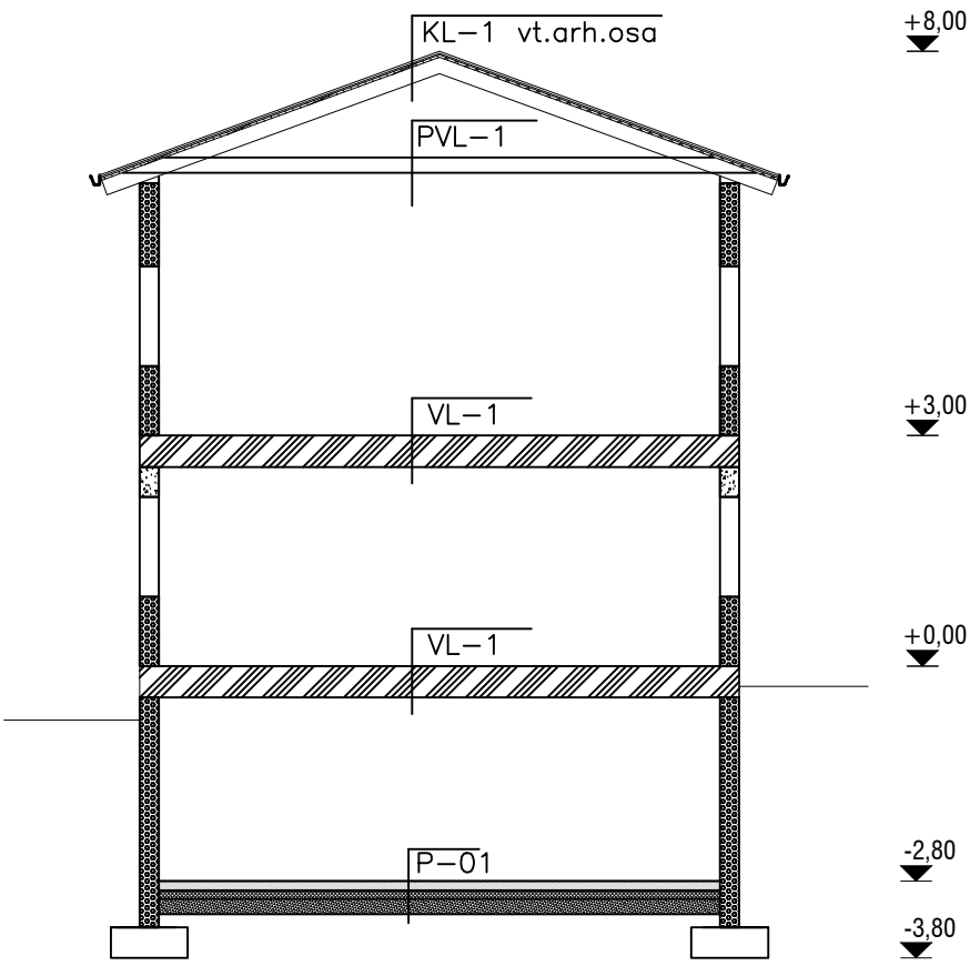
Lõige 2-2
