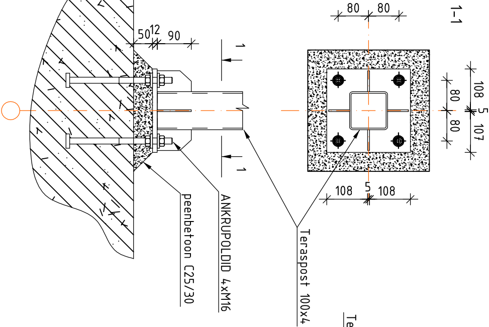
sõlm s3 1:20
