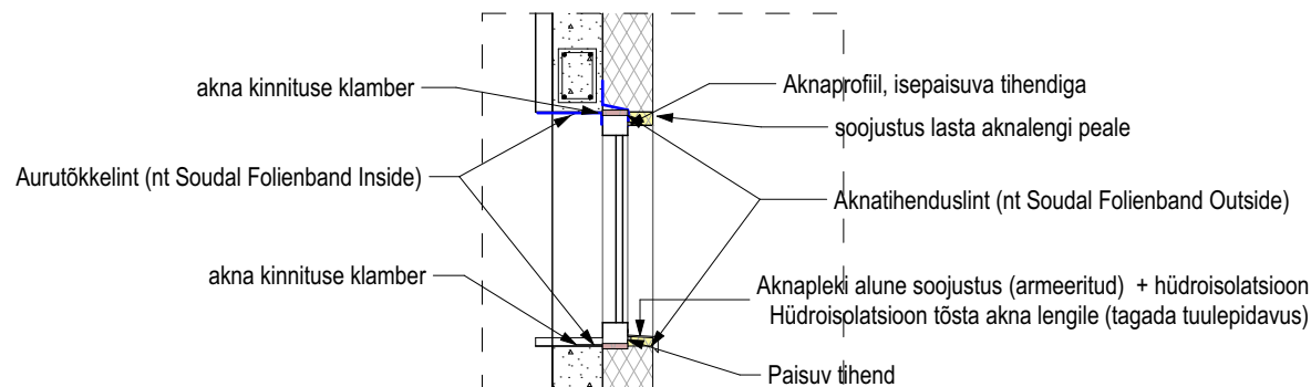
D-2 Aakna sõlm 1:25
