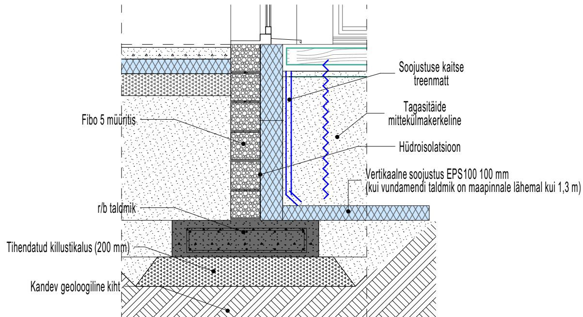
D-1 Sokkel 1:25
