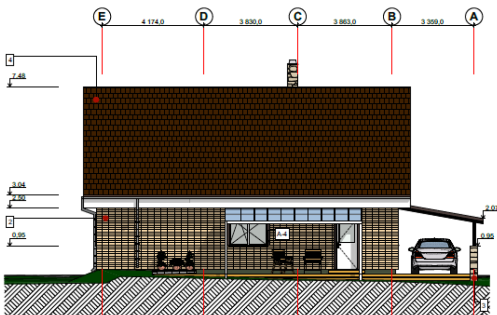
Vaade läänest
