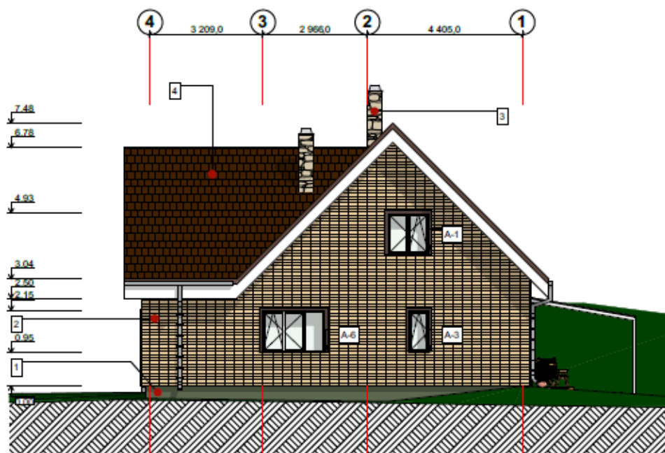
Vaade põhjast
