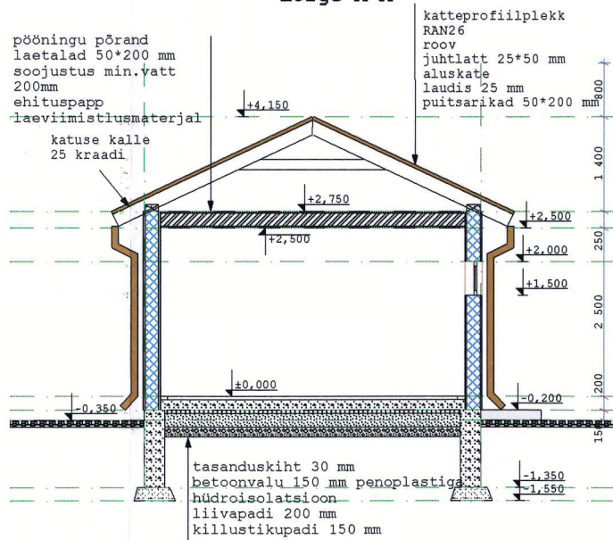
Lõige A-A
