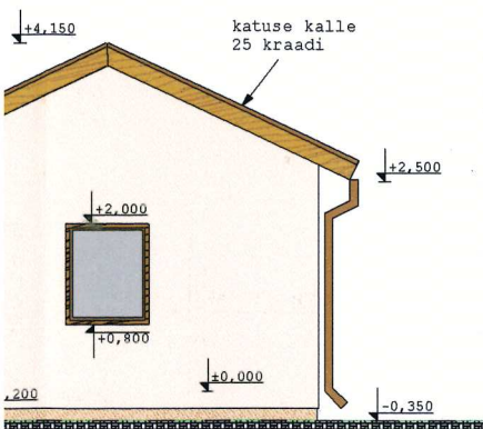
Vaade lõunast
