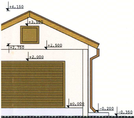
Vaade lõunast
