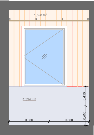
Lõige 4-4
