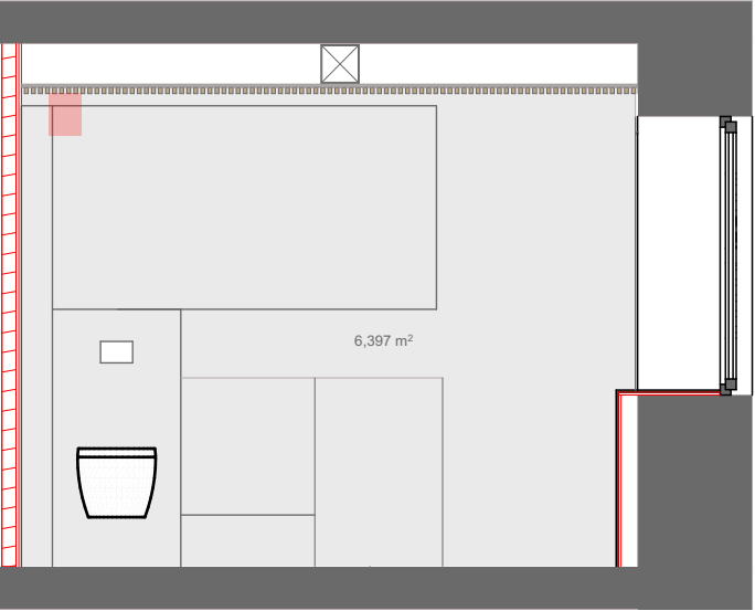
Lõige 1-1
