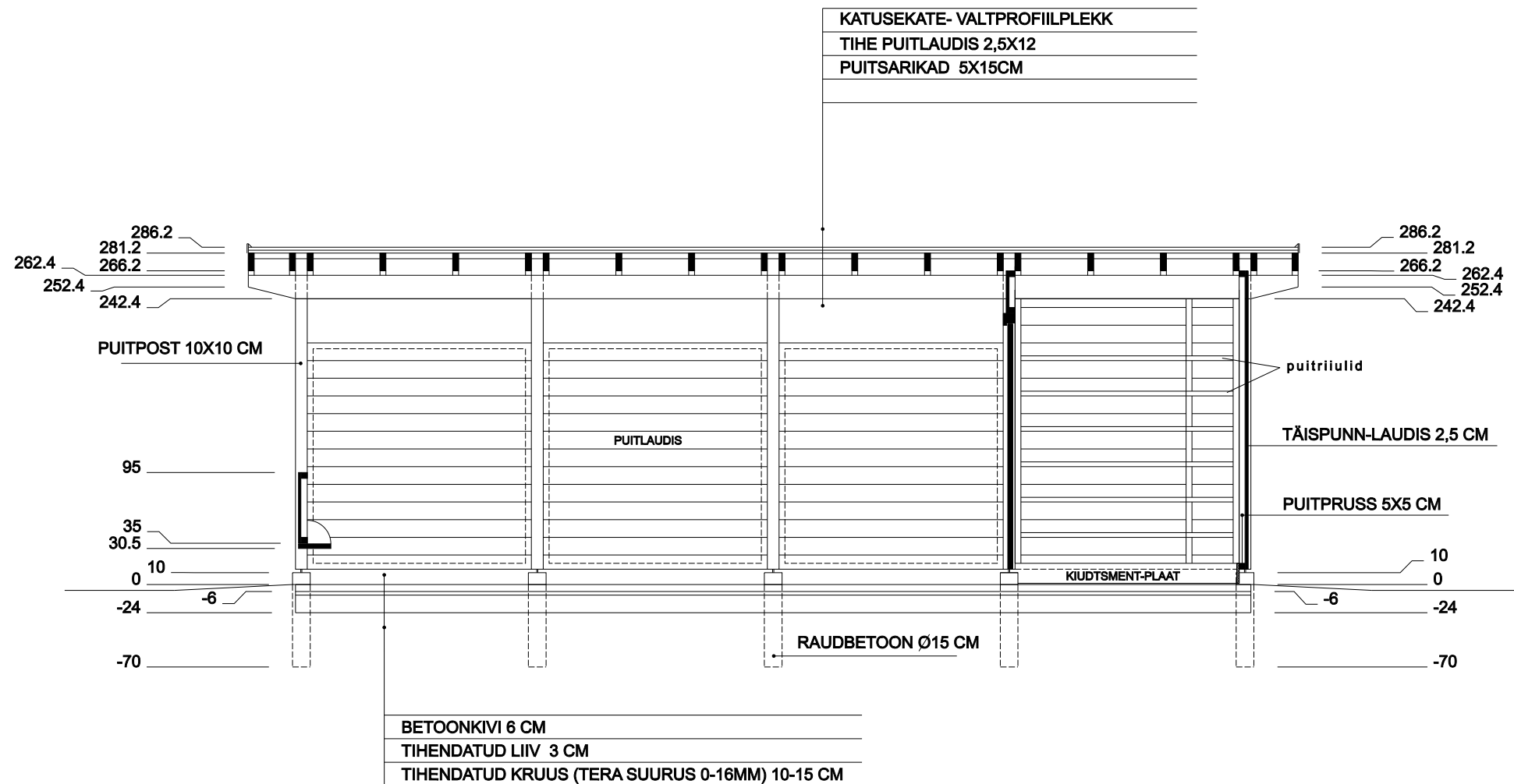
LÕIGE A-A M 1:50
