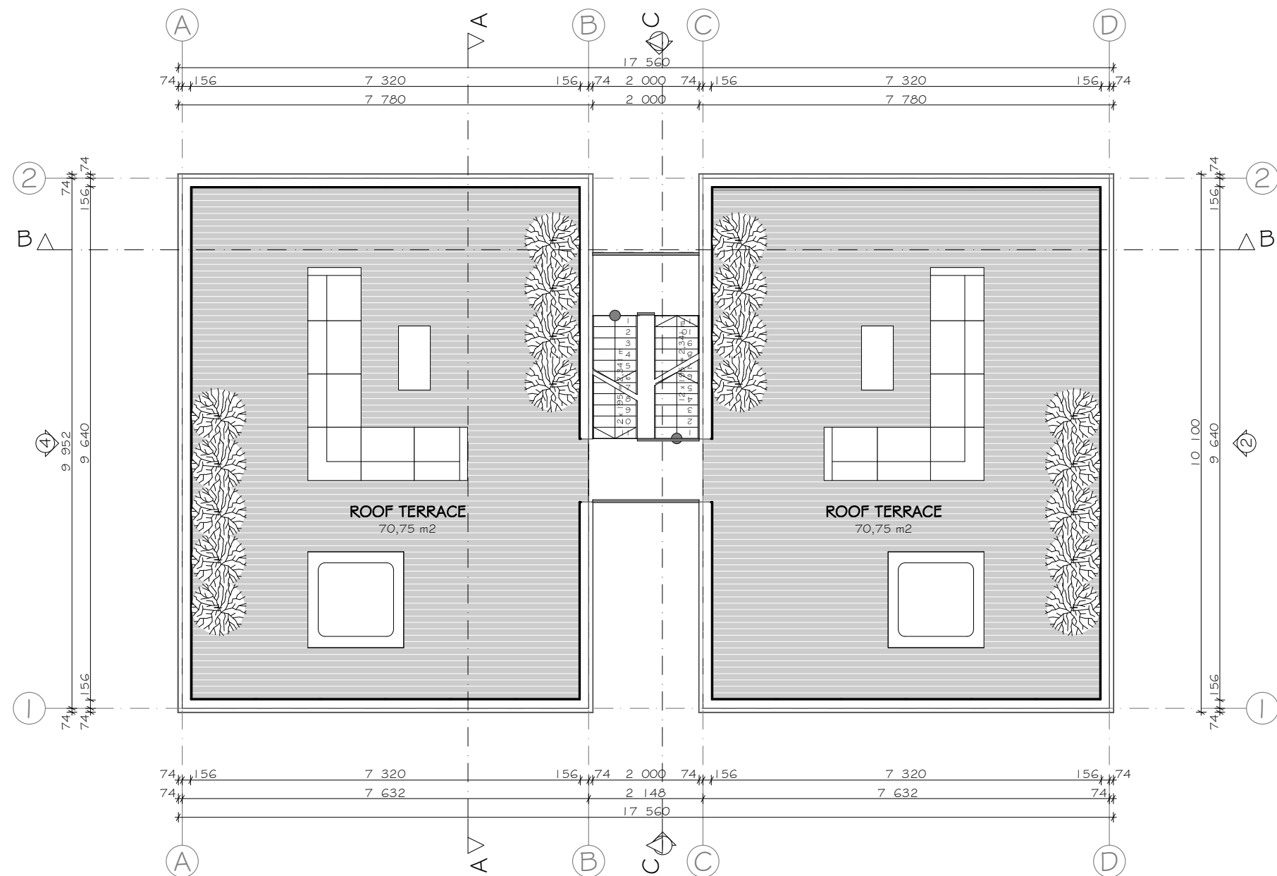
3 Plan 3. TAK 1:100
