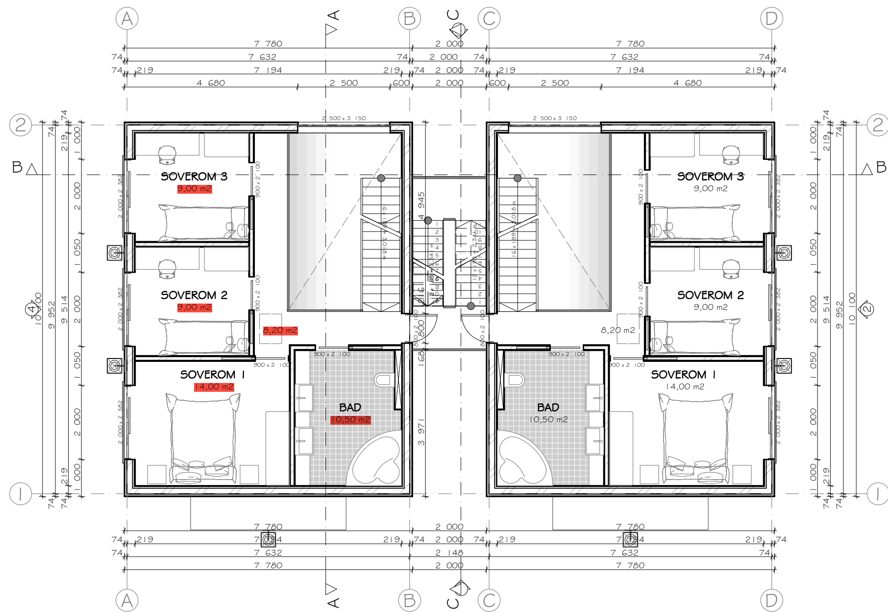
2 PLAN 2. ETASJE 1:100
