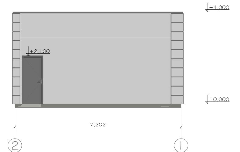
4 Elevation 1:100
