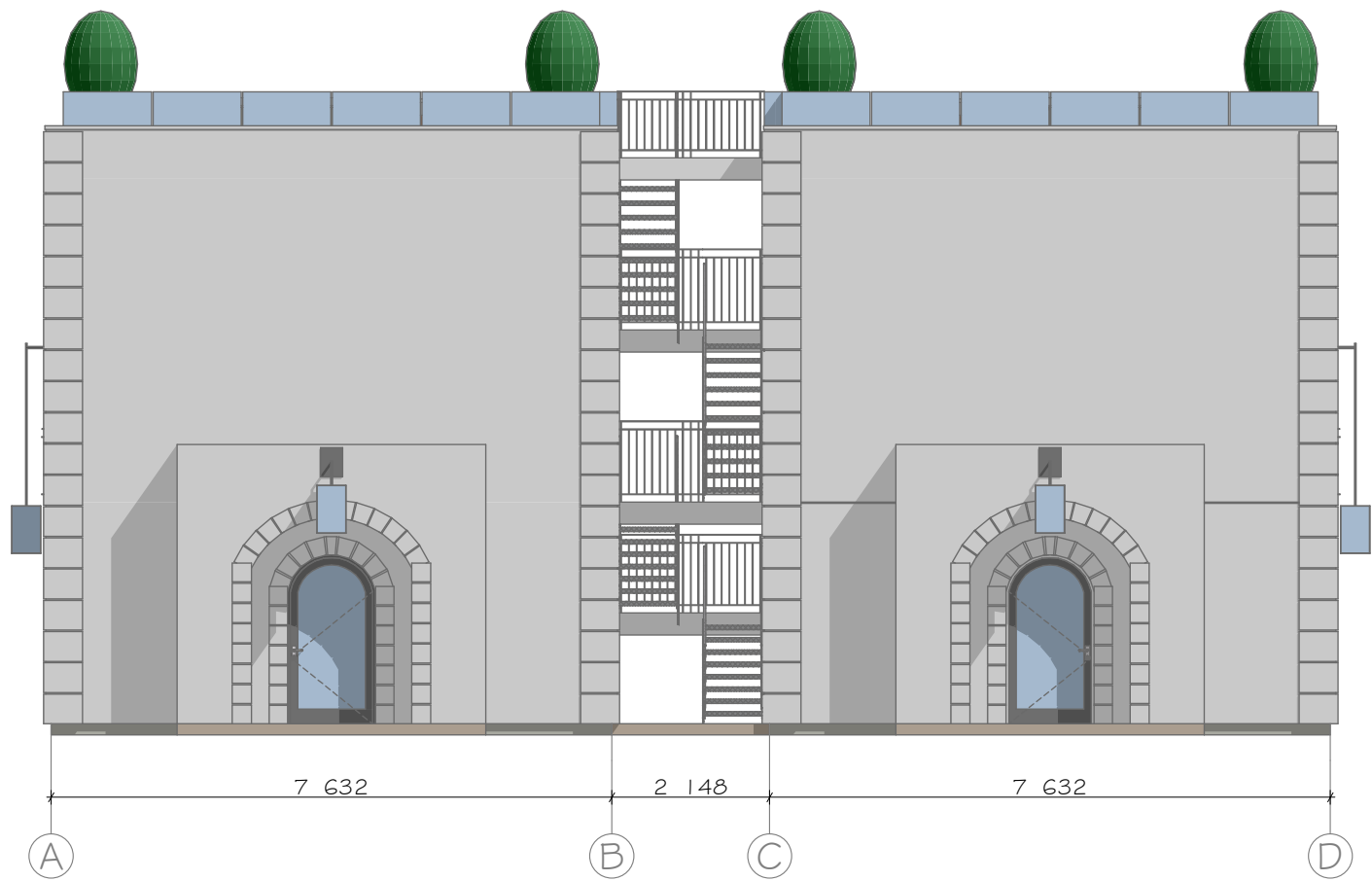
1 Elevation 1:100
