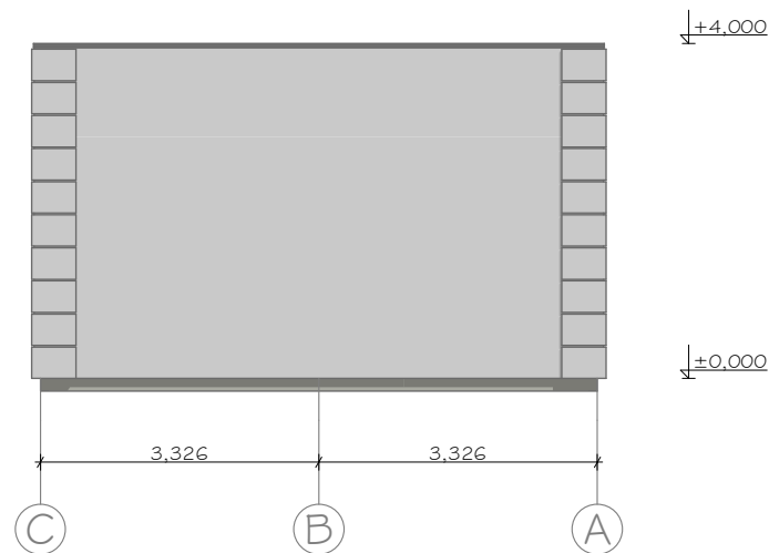
3 Elevation 1:100
