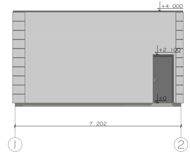
2 Elevation 1:100
