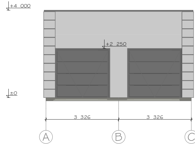
1 Elevation 1:100
