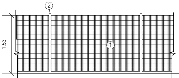
PIIRDEAIA VAATE FRAGMENT M1:50
