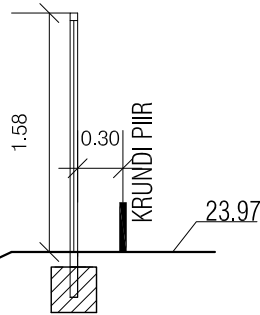
LÕIGE 1-1 M1:50
