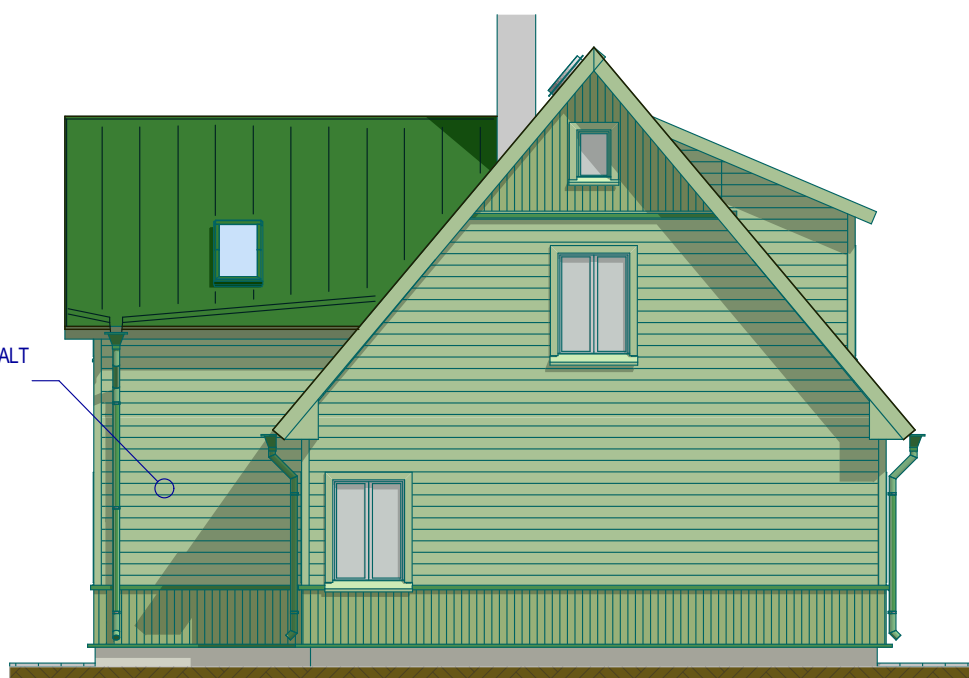
VAADE LÄÄNEST
