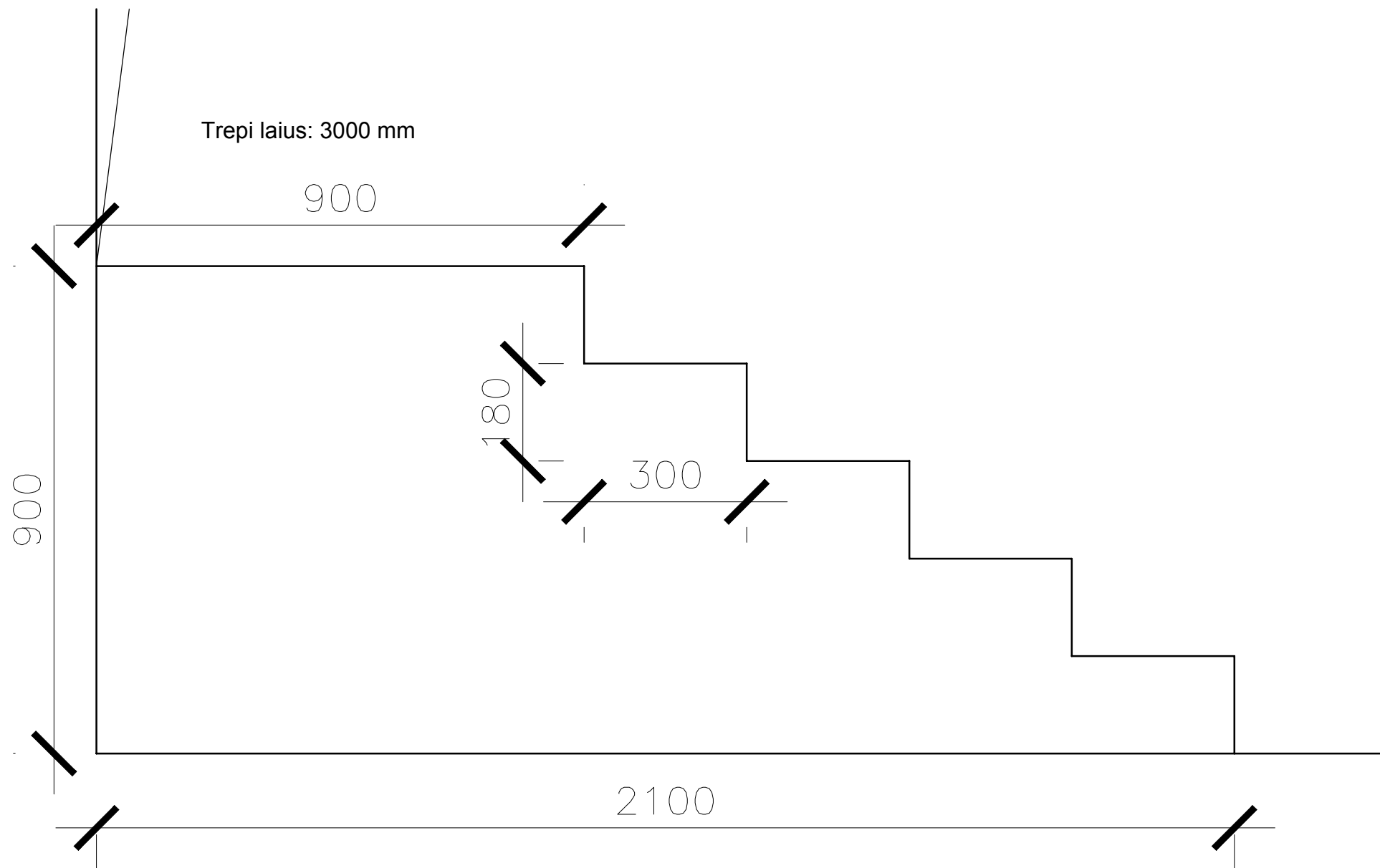
Pesubetoonist astmetega trepp M 1:10
