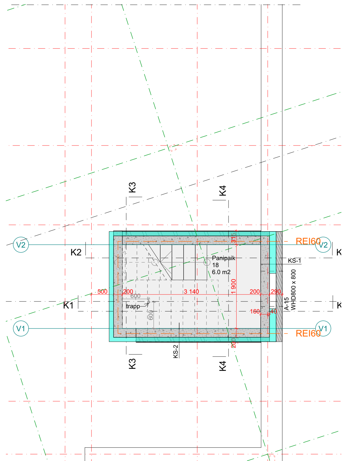
-1. Kelder (2) 1:50
