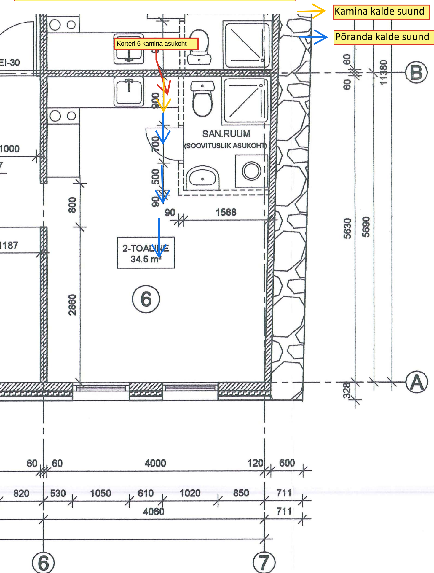
Lisa 3. Väljavõte 2004.aasta rekonstrueerimisprojekti 2.korruse plaanist
