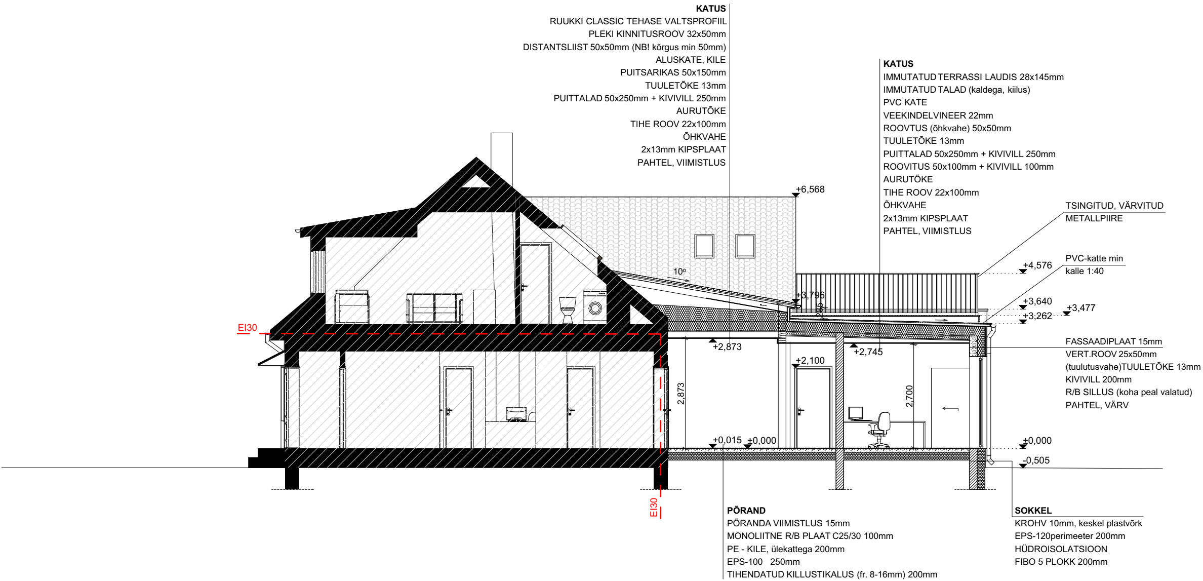
LÕIGE Y-Y
